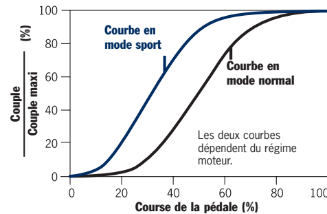
Courbes comparatives de l'accélérateur électronique en mode « Normal » et « Sport »
